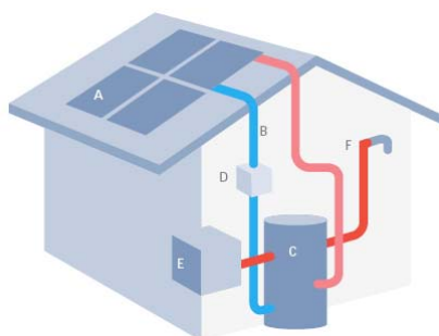
A. Sonnenkollektor B. Zirkulationsleitung C. Speicher D. Pumpe E. Zusatzheizung F. Zapfstelle für Warmwasser
